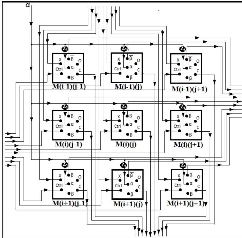
Fig. 8. CAM Array
