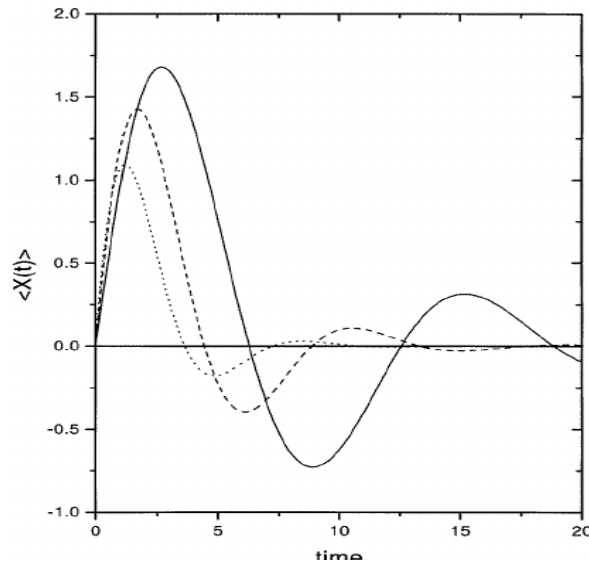
Fig. 7. Poisson noise
