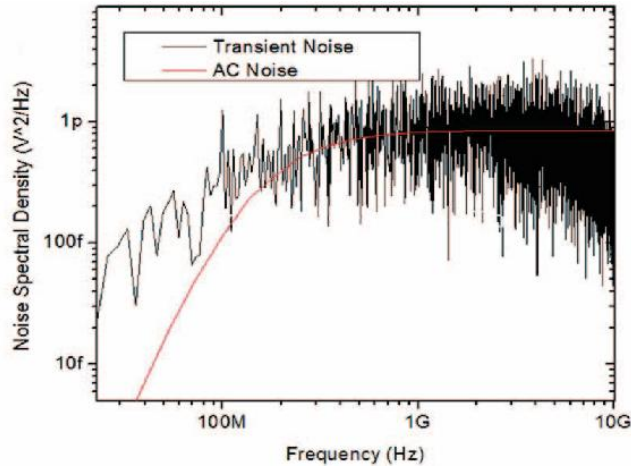
Fig. 8. Transient noise
